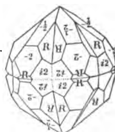
Chabazite.
